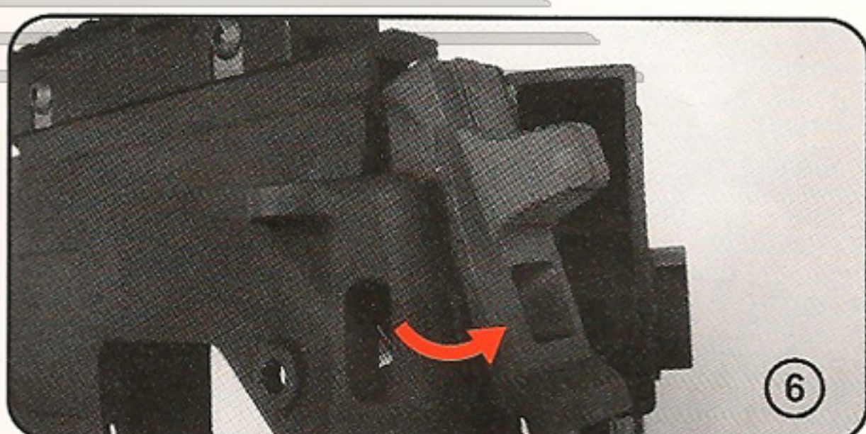
取下覆進簧頂塊
